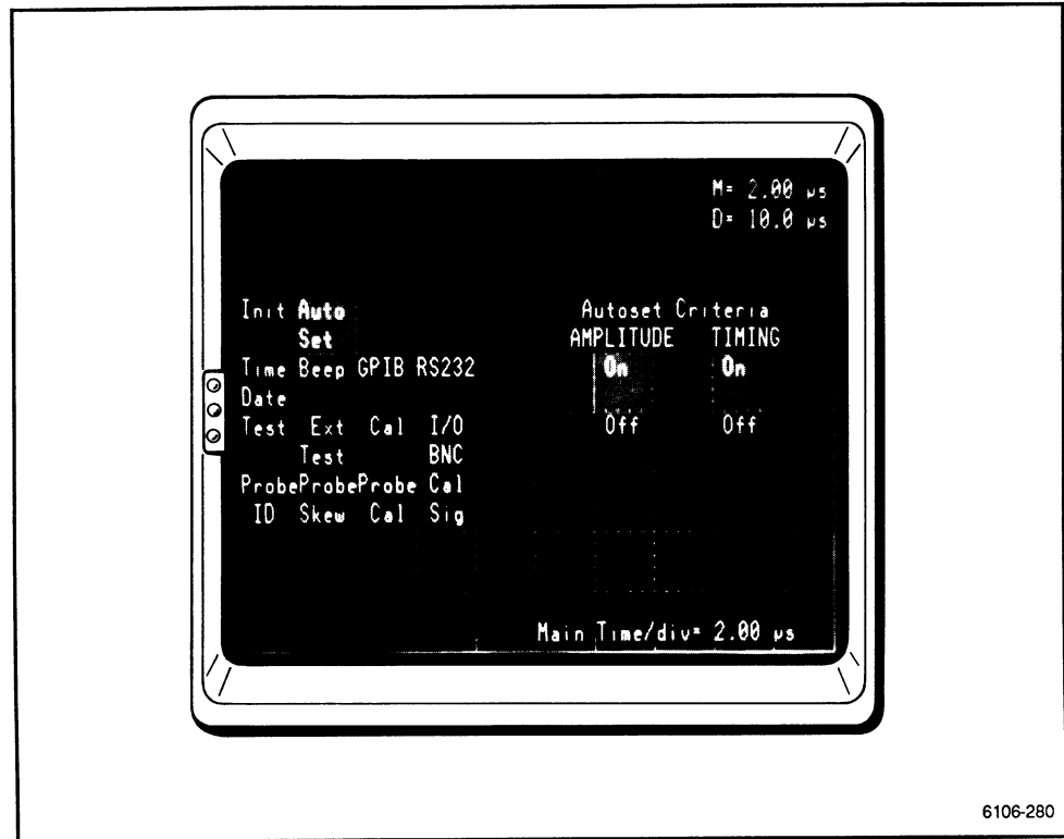
Figure 2-81. Autoset menu.
