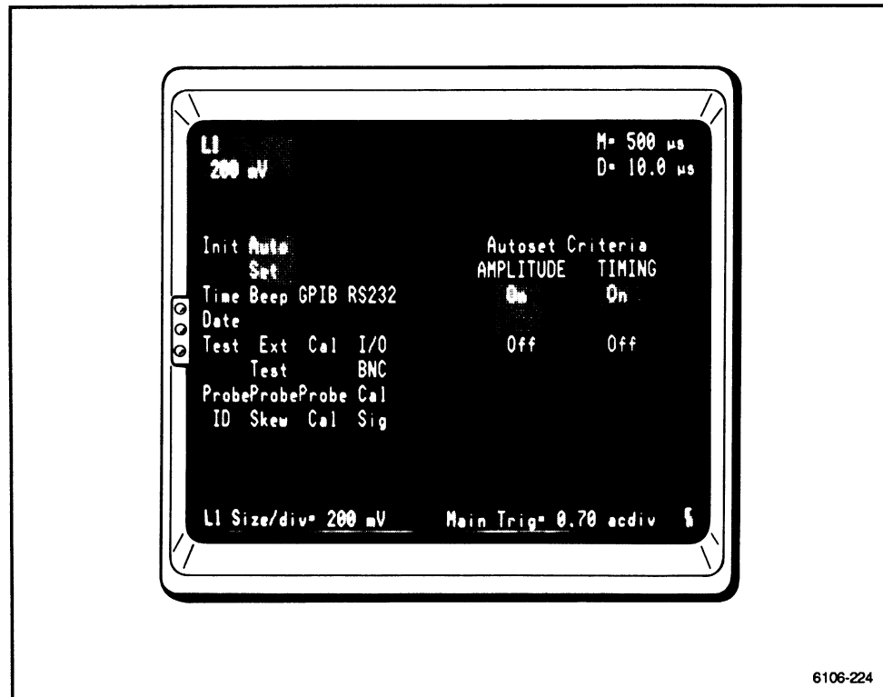
Figure 2-26. Autoset menu.
